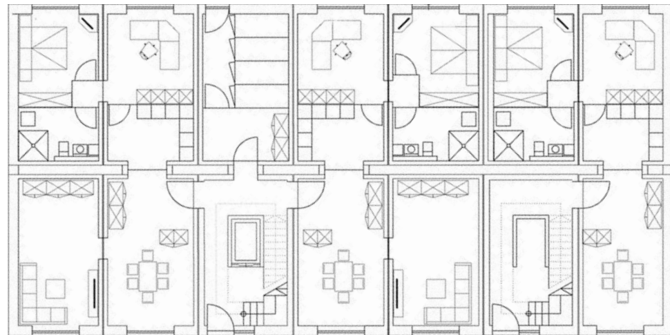
GRUNDRISS EG
