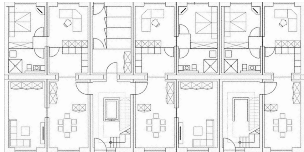
GRUNDRISS 1. OG
