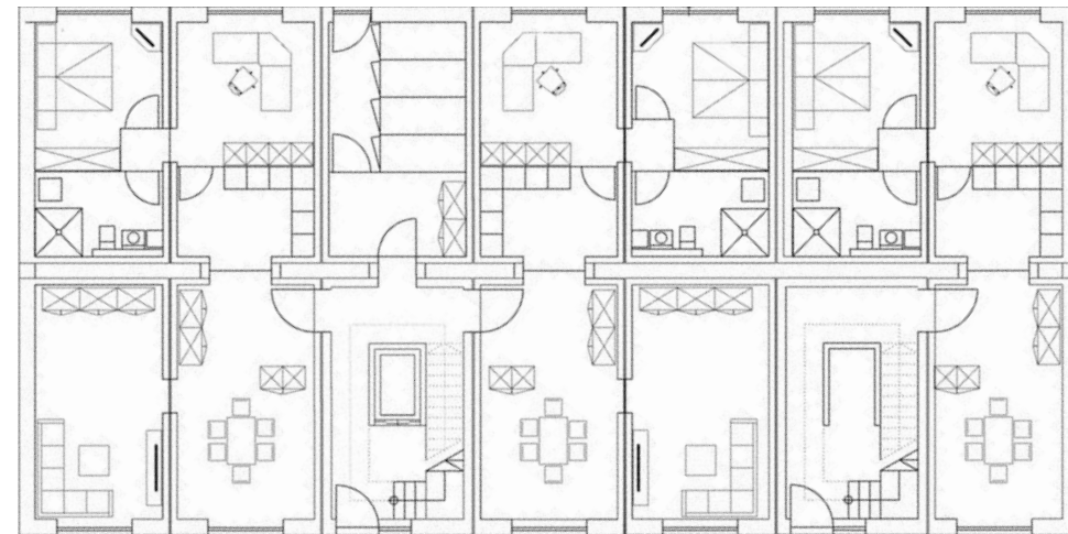
GRUNDRISS 2. OG
